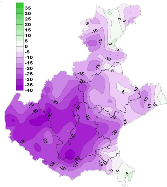
Scarto % precipitazione media 2017 rispetto alla media 1993-2016
